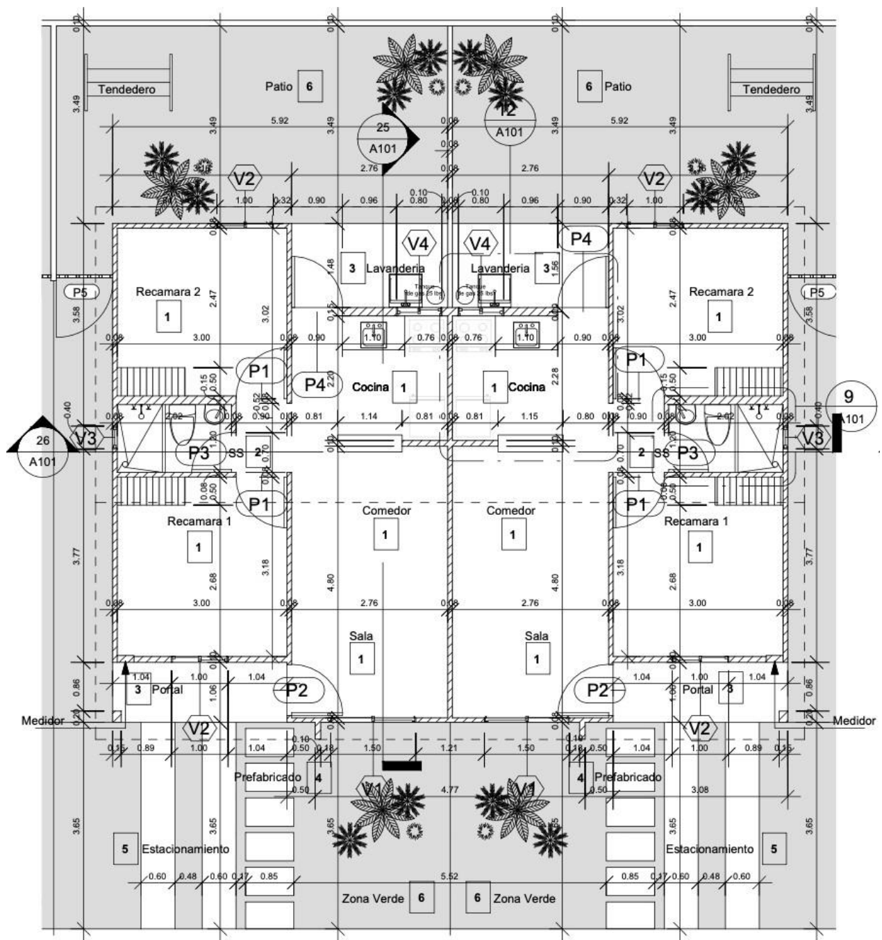
1 Planta Arquitectonica 1 : 75
